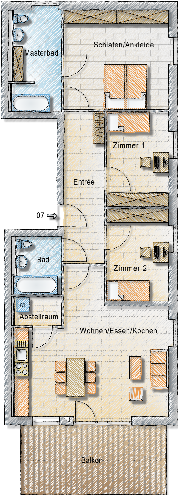
2 Obergeschoss
